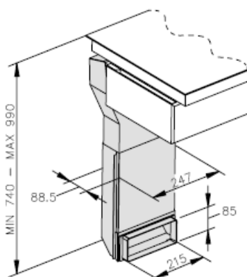
Uscita a zoccolo Plinth outlet
